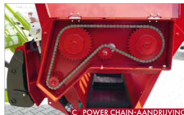
C POWER CHAIN-AANDRIJVING
